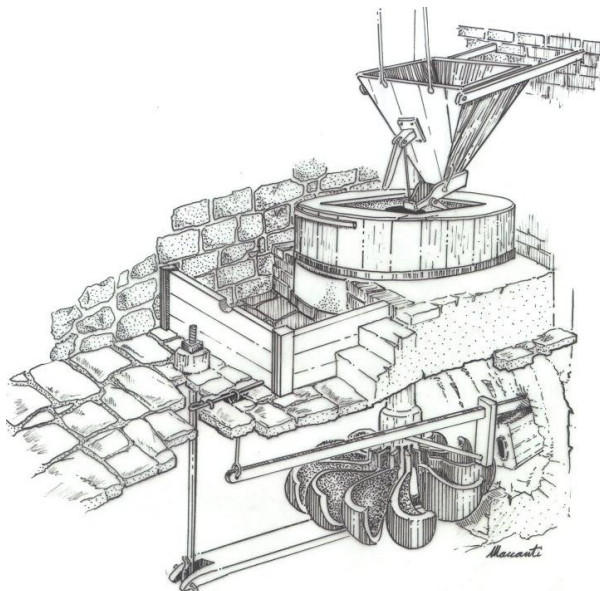
Principskiss på skvaltkvarnens funktionssätt.
